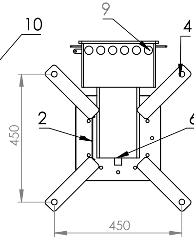
B-VIEW
